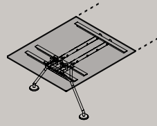
Rectangular end top for meeting table Piano terminale rettangolare per tavolo meeting L×W 140×120 / 160×120 / 180×120 / 200×120 / 160×140 / 200×140 cm, H 72 cm L×W 55 ¼×47 ½ / 63×47 ½ / 70 ¾×47 ½ / 78 ¾×47 ½ / 63×55 ¼ / 78 ¾×55 ¼ ", H 28 ½ "
